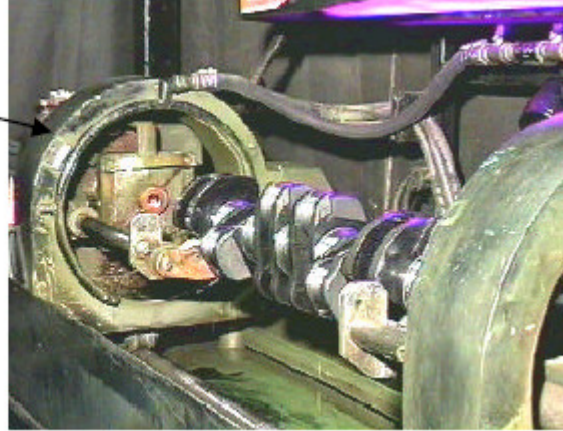
Figura 20 - Ensaio de um virabrequim pela técnica da bobina
