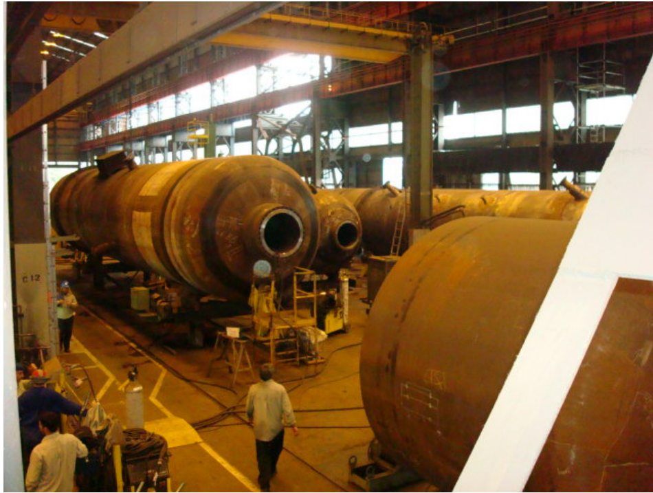
Figura 6 - Caldeiraria pesada - Confab Equipamentos
