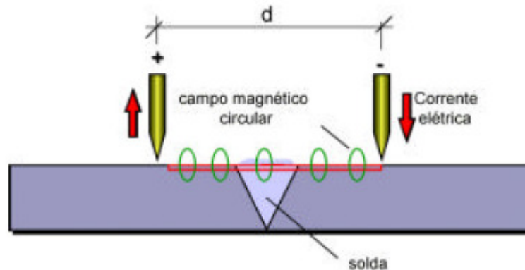
Figura 19 - Esquematização da técnica dos eletrodos
