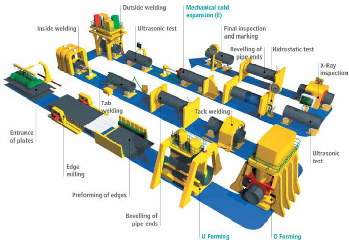
Figura 4 - Processo de manufatura de tubos pelo método U-O-E
